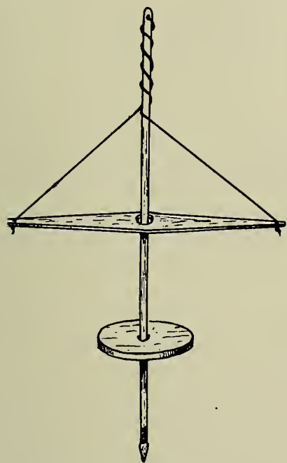
FIG. 46.—Pump drill.
