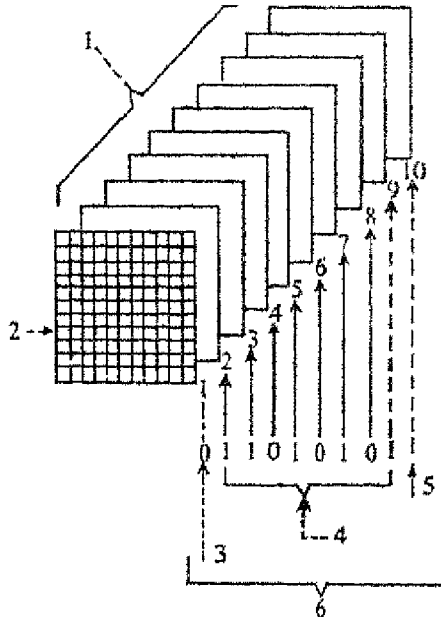
चित्र 6.4 : फ़ैराइट कोर व्यवस्था
